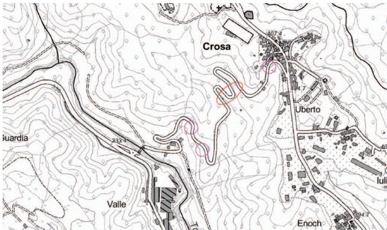
Localizzazione intervento su carta BDTRE in rosso dissesto principale con asportazione infrastruttura, in magenta ulteriori cedimenti
